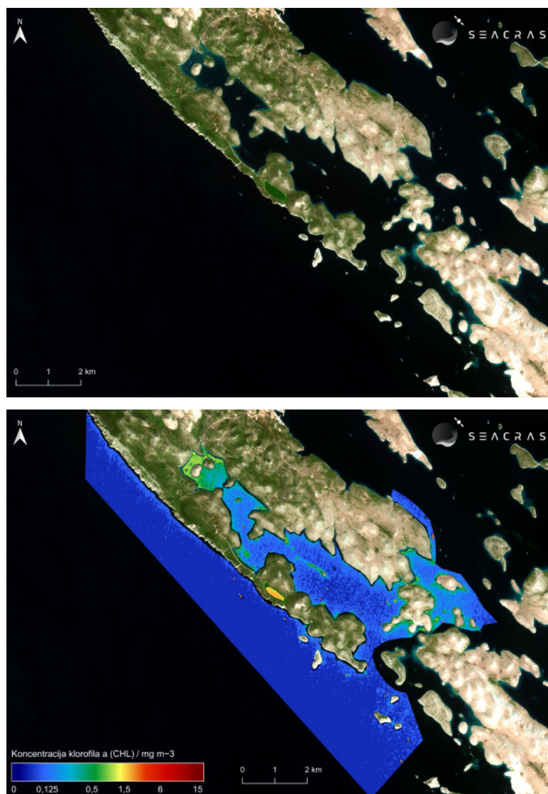
Slika 6. Panel sa satelitskom snimkom u RGB formatu (gore), te obrađenom snimkom na kojoj je kartirana vrijednost koncentracije klorofila a za područje Parka prirode Telašćica (dolje) na datum 24.08.2024.
