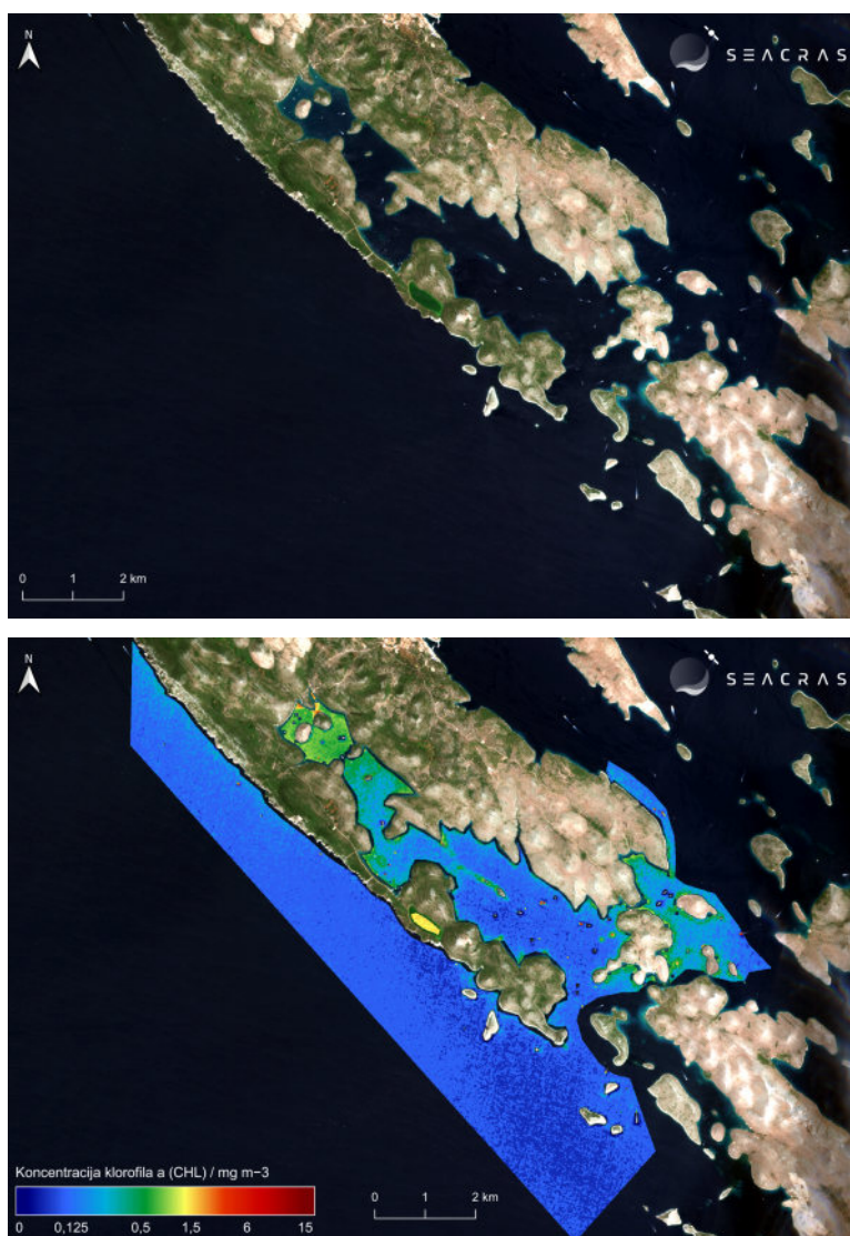
Slika 3. Panel sa satelitskom snimkom u RGB formatu (gore), te obrađenom snimkom na kojoj je kartirana vrijednost koncentracije klorofila \alpha za područje Parka prirode Telašćica (dolje) na datum 04.08.2024.
