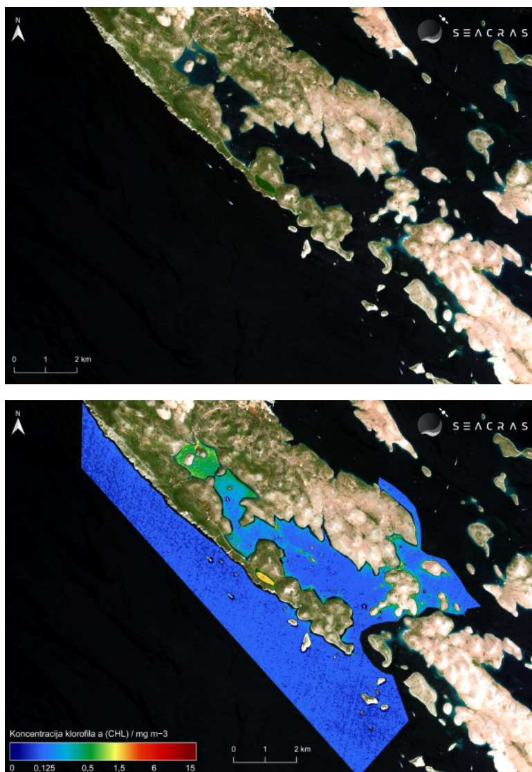
Slika 4. Panel sa satelitskom snimkom u RGB formatu (gore), te obrađenom snimkom na kojoj je kartirana vrijednost koncentracije klorofila a za područje Parka prirode Telašćica (dolje) na datum 09.08.2024.
