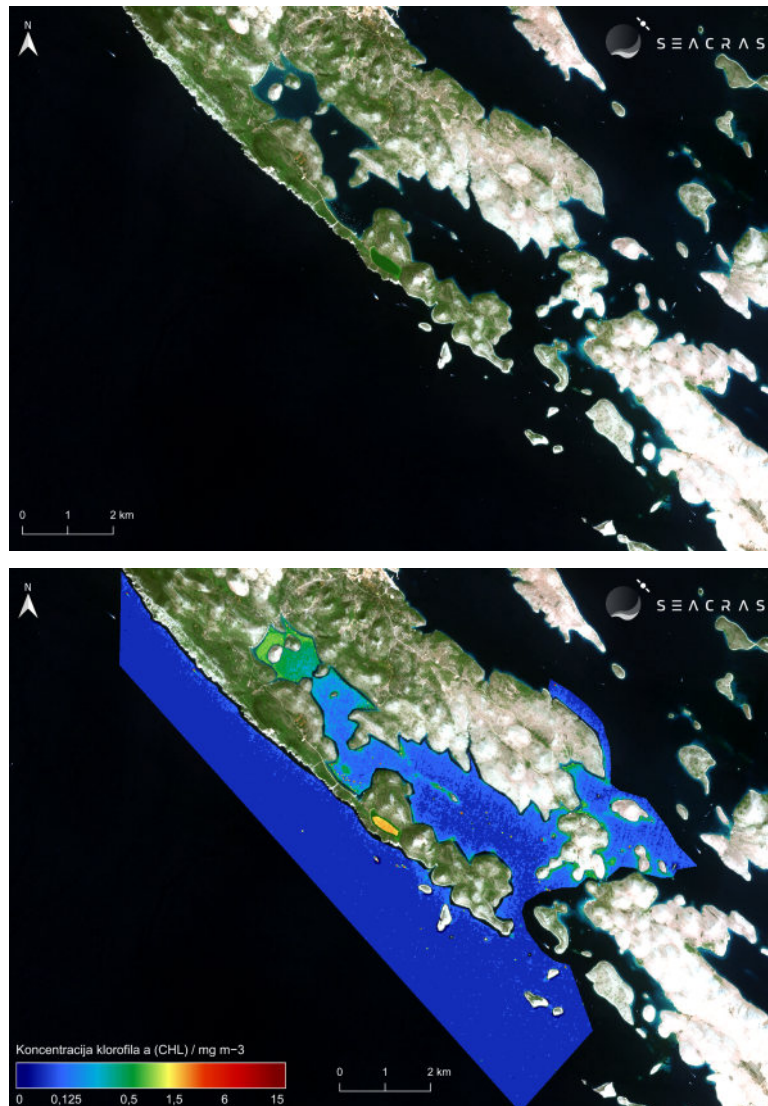
Slika 7. Panel sa satelitskom snimkom u RGB formatu (gore), te obrađenom snimkom na kojoj je kartirana vrijednost koncentracije klorofila a za područje Parka prirode Telašćica (dolje) na datum 29.08.2024.
