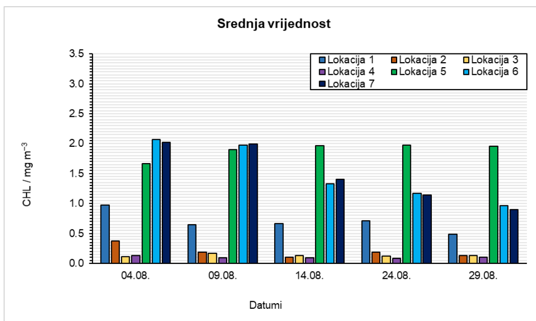
Slika 10. Stupčasti grafikon s prikazom srednje vrijednosti koncentracije klorofila a na Lokacijama 1 - 7 za sve datume u kolovozu 2024.
