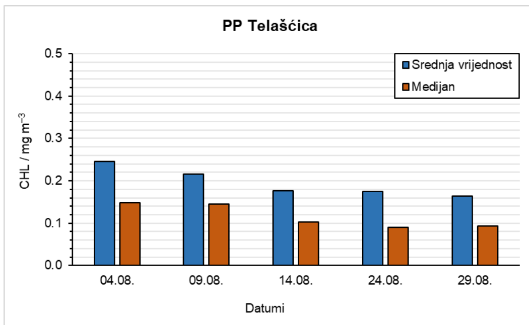
Slika 9. Stupčasti grafikon s prikazom srednje vrijednosti i medijana koncentracije klorofila a za sve datume u kolovozu 2024.
